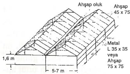
Şekil 1: Beşik çatılı sera
