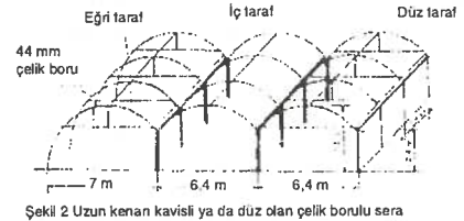
Şekil 2: Uzun kenar kavisli ya da düz olan çelik borulu sera
