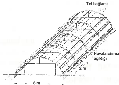
Şekil 3: Sürekli havalandırılmalı yay çatılı tünel sera
